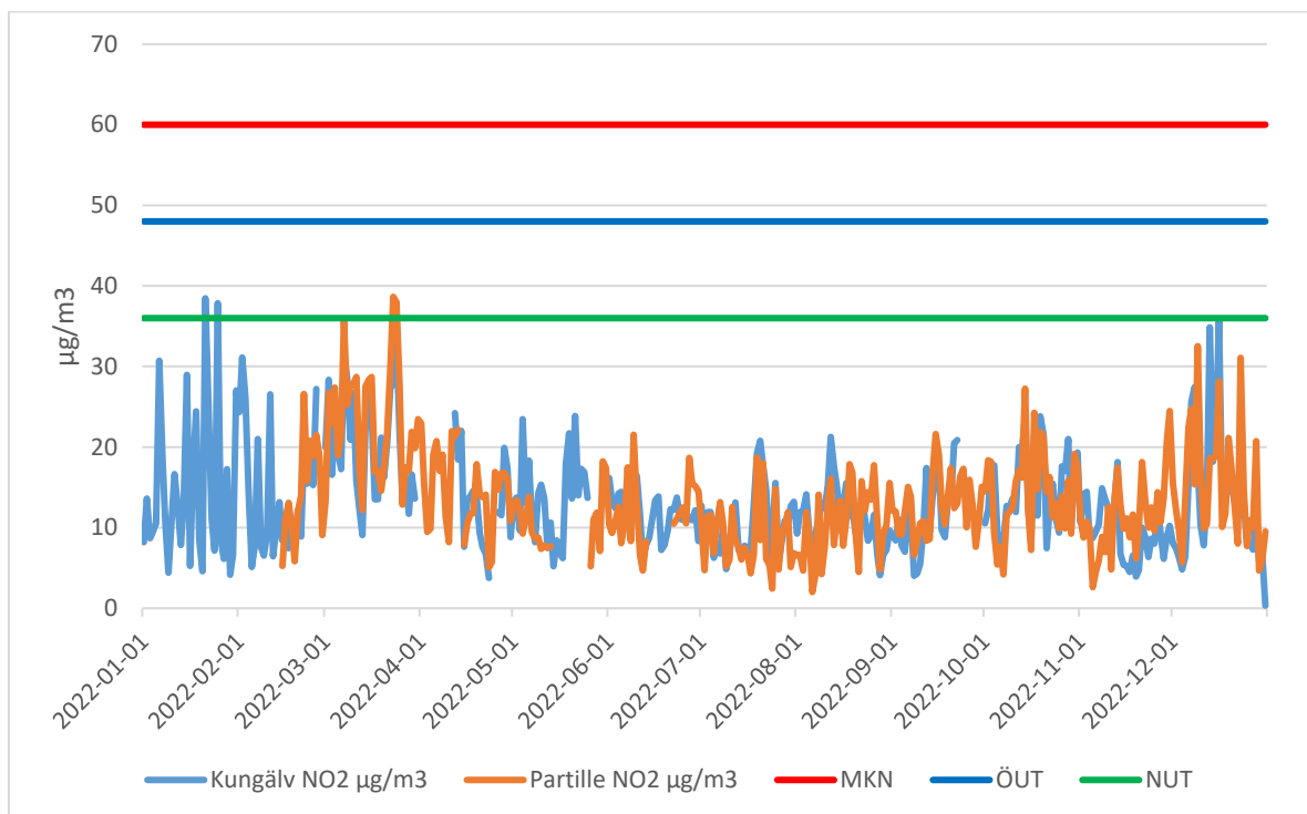
Figur4 Dygnsmedelvärden av kvävedioxidhalter under ett år i gaturum i Kungälv och Partille under 2022.
