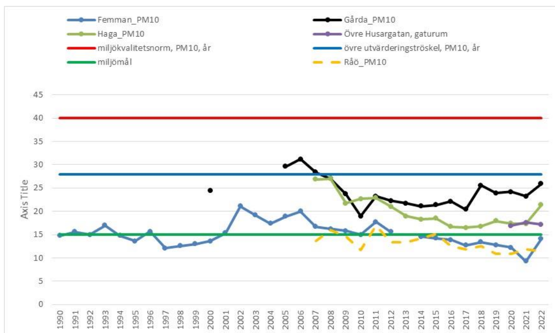
Figur 5. Årsmedelvärden (1990 – 2022) av partiklar (PM 10 ) vid kontinuerliga mätstationer i Göteborg samt vid den nationella bakgrundsstationen Råö (Rörvik t.om 2001) utanför Kungsbacka.
