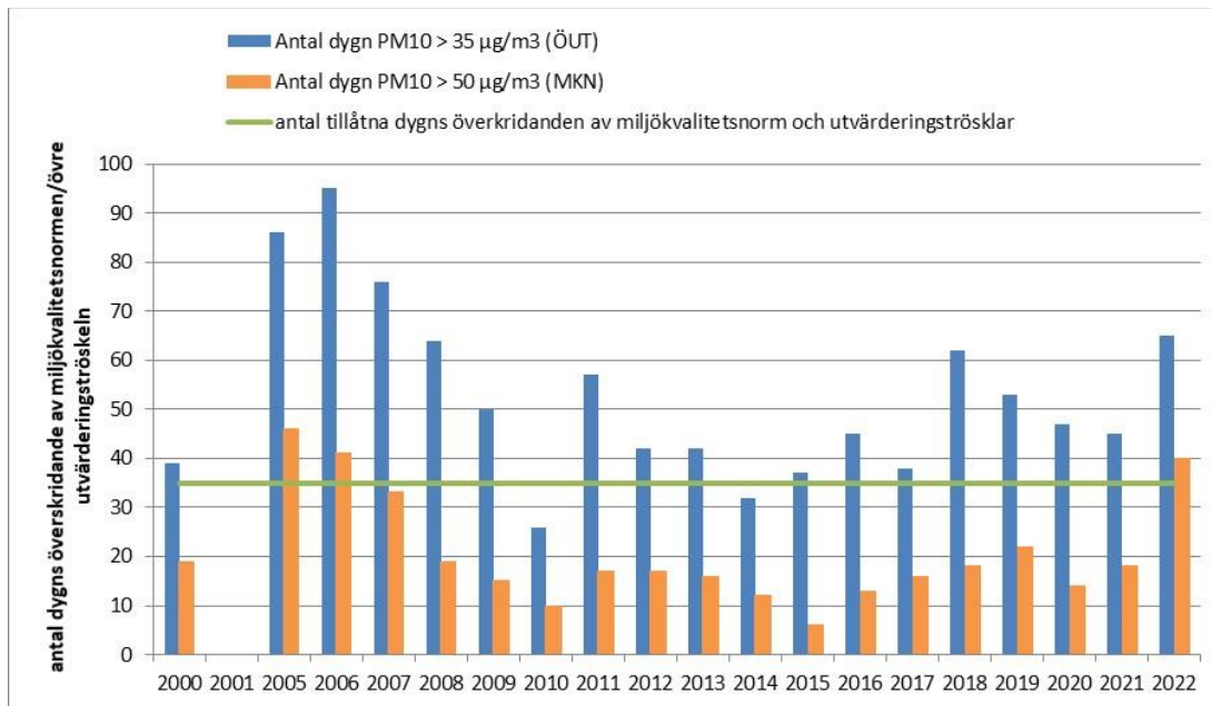
Figur 6. Antal dygns överskridanden av miljö kvalitetsnormen och övre utvärderingströskeln för dygnsmedelvärden av PM 10 . Resultat från mätningar under åren 2000 – 2022 vid mätstationen i Gårda.
