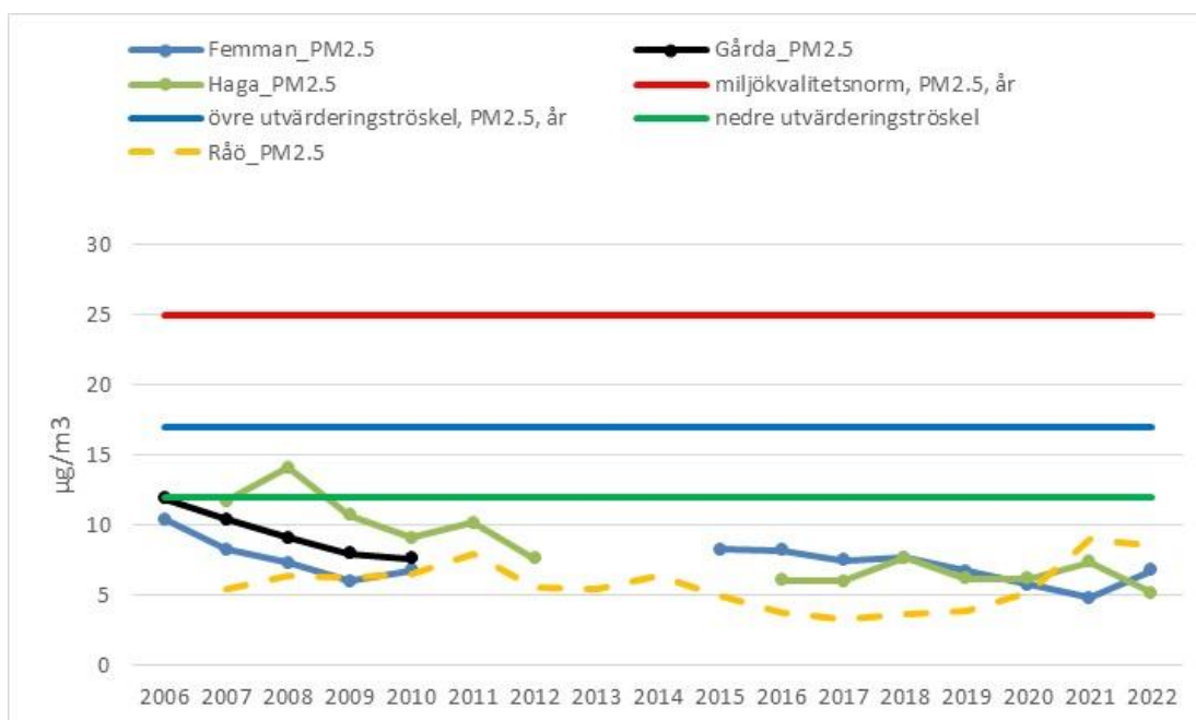
Figur 7. Årsmedelvärden av partiklar (PM 2.5 ) vid kontinuerliga mätstationer i Göteborg samt vid den nationella bakgrundsstationen Råö (Rörvik t.om 2001) utanför Kungsbacka.
