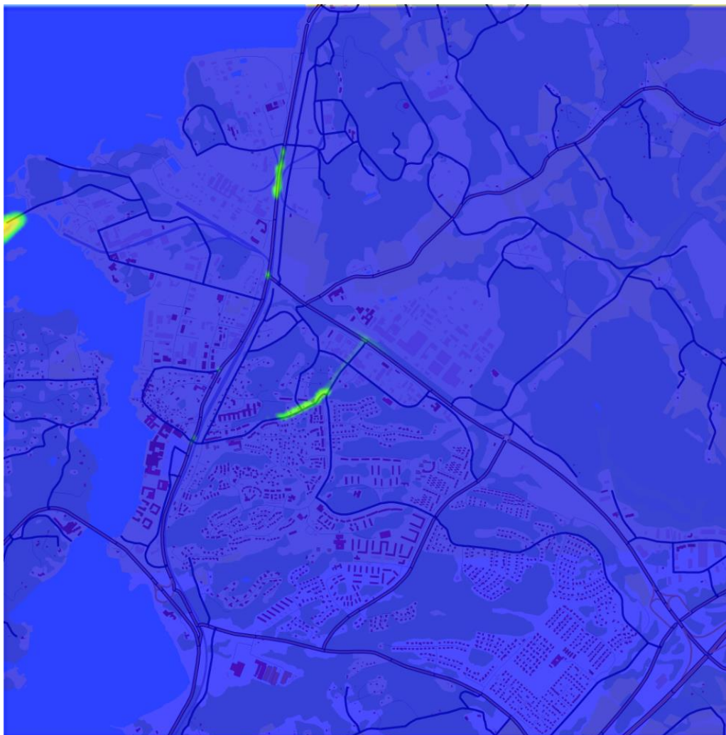
Figur 1. Beräknat årsmedelvärde för kvävedioxidhalter i Stenungsund tätort i Stenungsunds kommun år 2015.
