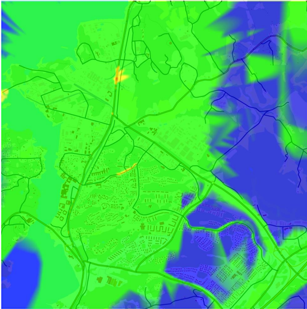
Figur 3. Beräknat timmedelvärde (98-percentil) för kvävedioxidhalter i Stenungsund tätort i Stenungsunds kommun år 2015.
