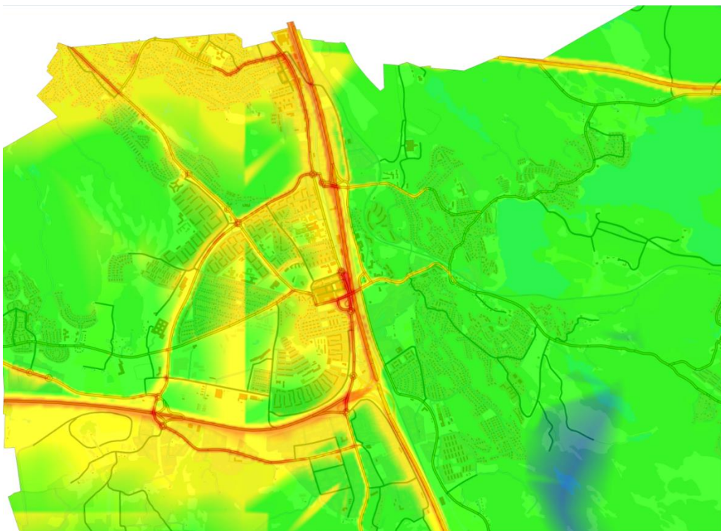
Figur 2. Beräknat dygnsmedelvärde (98-percentil) för kvävedioxidhalter i Mölndals tätort i Mölndals kommun år 2015.
