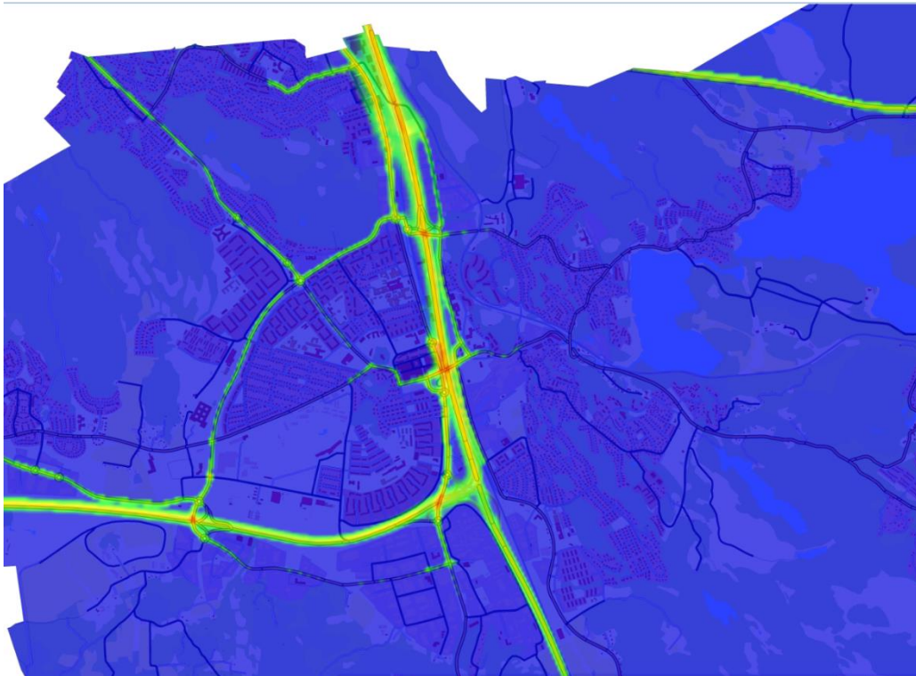
Figur 1. Beräknat årsmedelvärde för kvävedioxidhalter i Mölndals tätort i Mölndals kommun år 2015.
