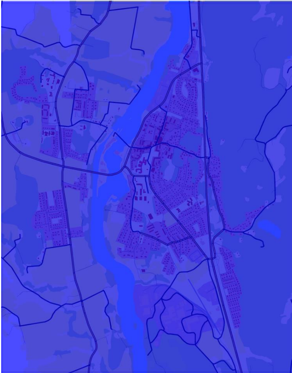
Figur 1. Beräknat årsmedelvärde för kvävedioxidhalter i Lilla Edets tätort i Lilla Edets kommun år 2015.
