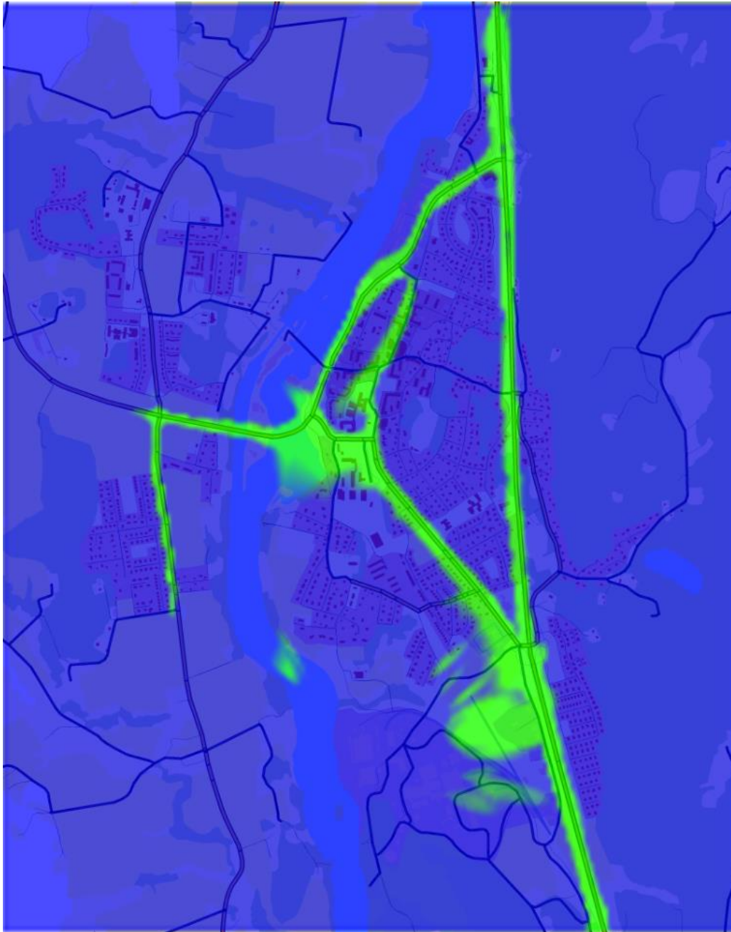
Figur 3. Beräknat timmedelvärde (98-percentil) för kvävedioxidhalter i Lilla Edets tätort i Lilla Edets kommun år 2015.
