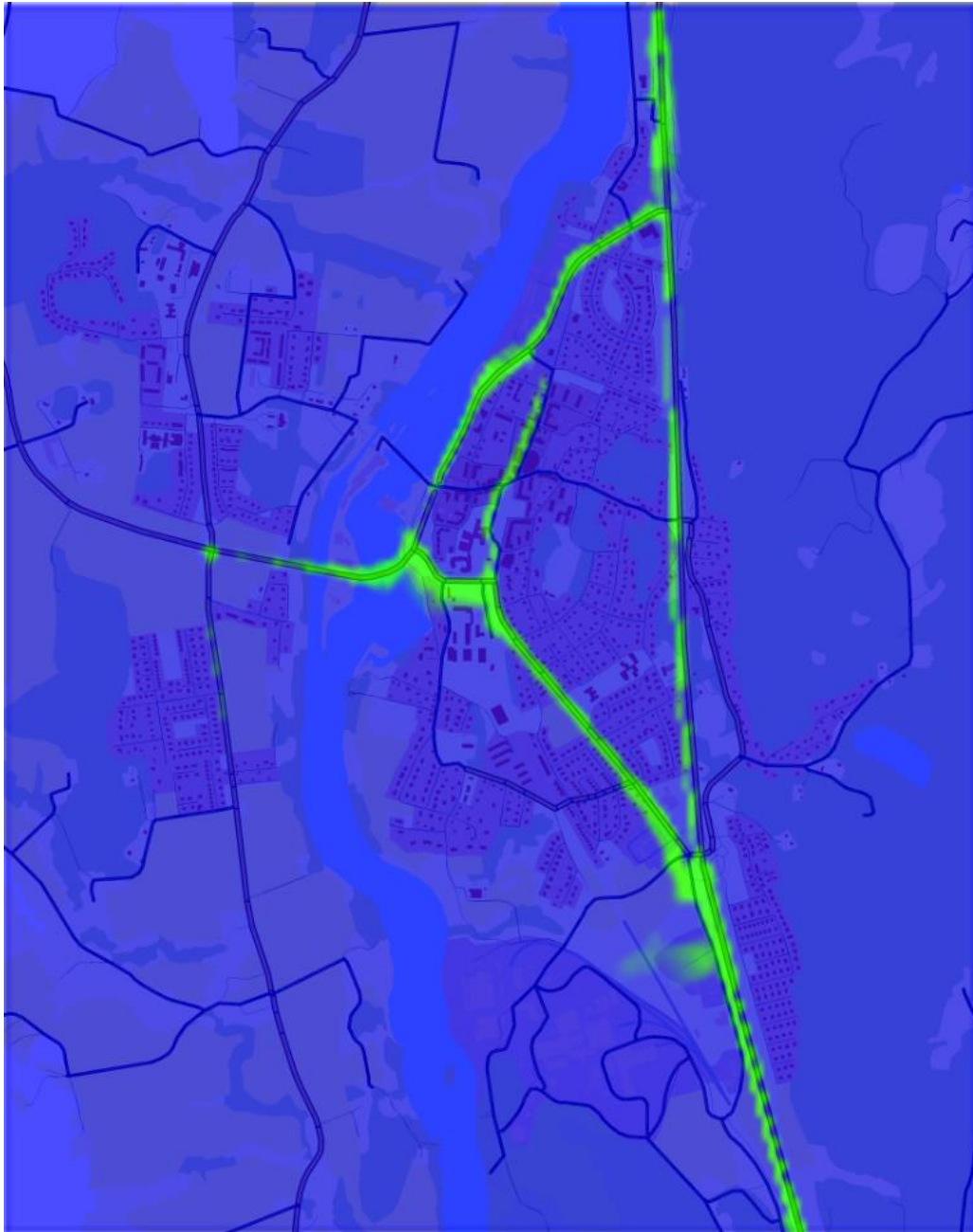
Figur 2. Beräknat dygnsmedelvärde (98-percentil) för kvävedioxidhalter i Lilla Edets tätort i Lilla Edets kommun år 2015.
