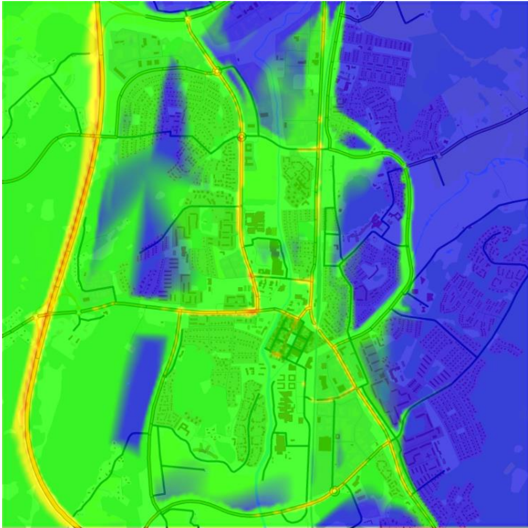
Figur 2. Beräknat dygnsmedelvärde (98-percentil) för kvävedioxidhalter i Kungsbacka tätort i Kungsbacka kommun år 2015.
